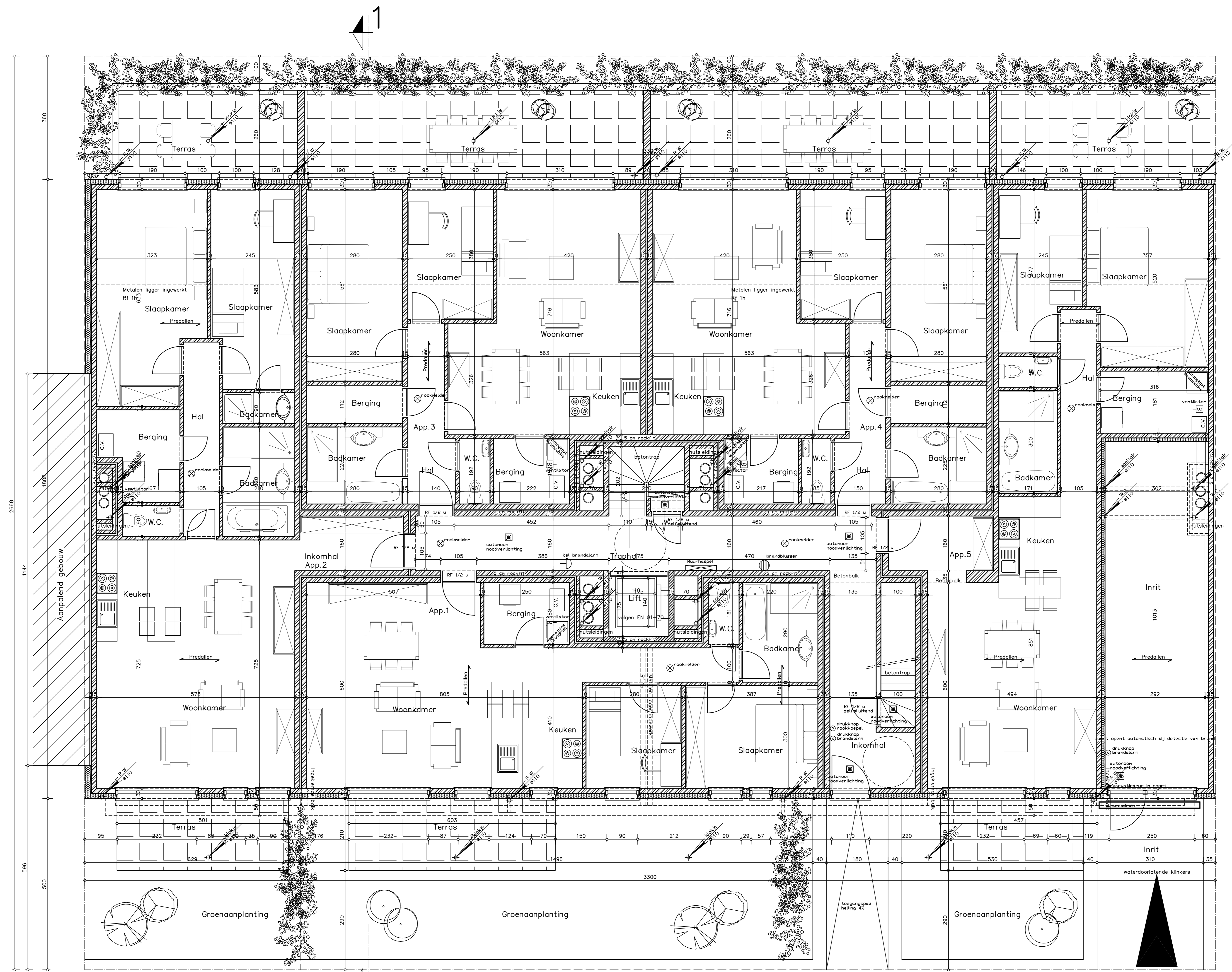
Gelijkvloers nivo +000
